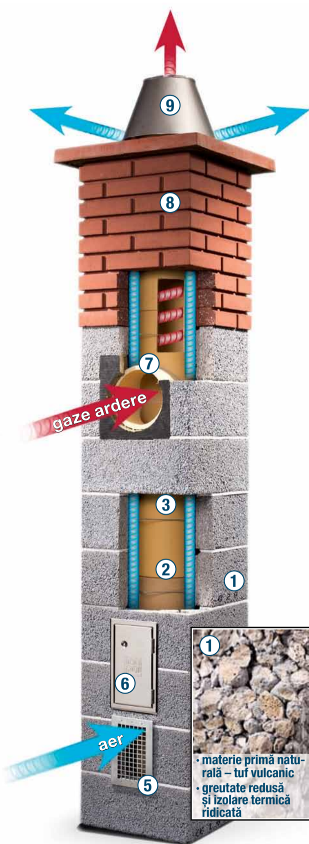
SPS zonă conectare cazan
